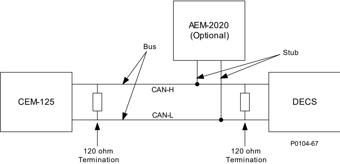
Figure 5-3. Interface du bus CAN avec le CEM-125 en procurant une extrémité du bus
