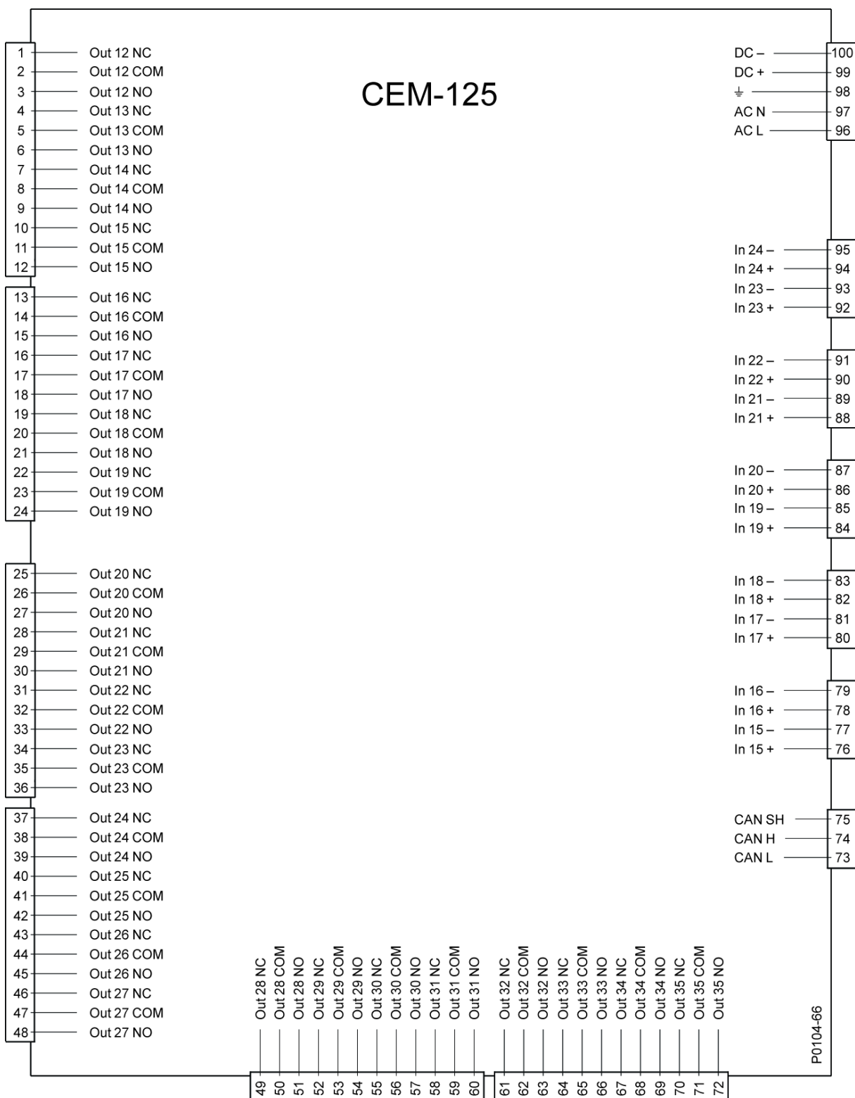
Figure 5-1. Bornes de contact du CEM-125
