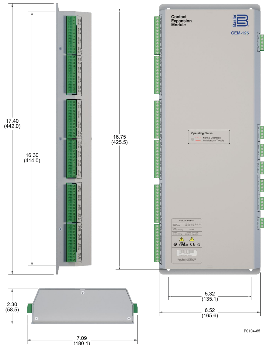
Abbildung 4-1. CEM-125 Gesamtabmessungen
