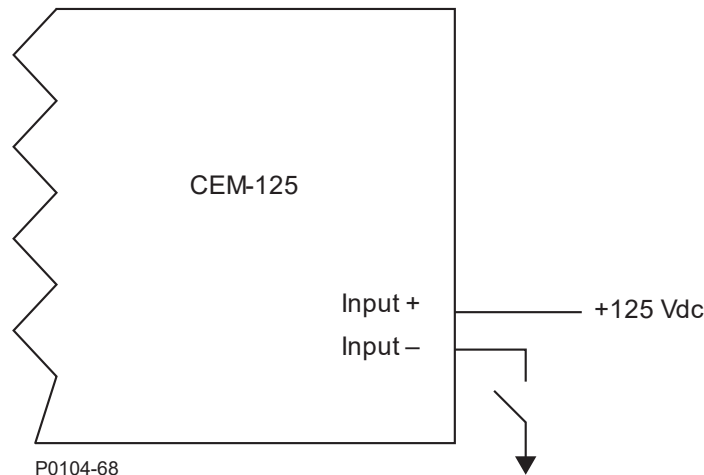
Abbildung 5-2. CEM-125 Klemmen
