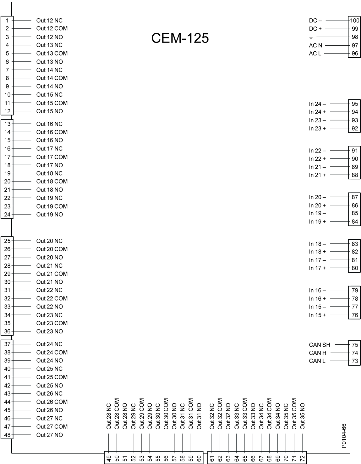
Figura 5-1. Terminales de contacto CEM-125
