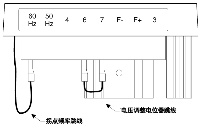
图2. 跳线位置
