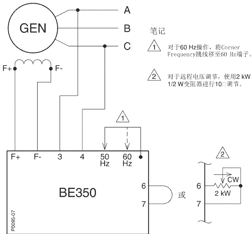
图5. 典型接线图
