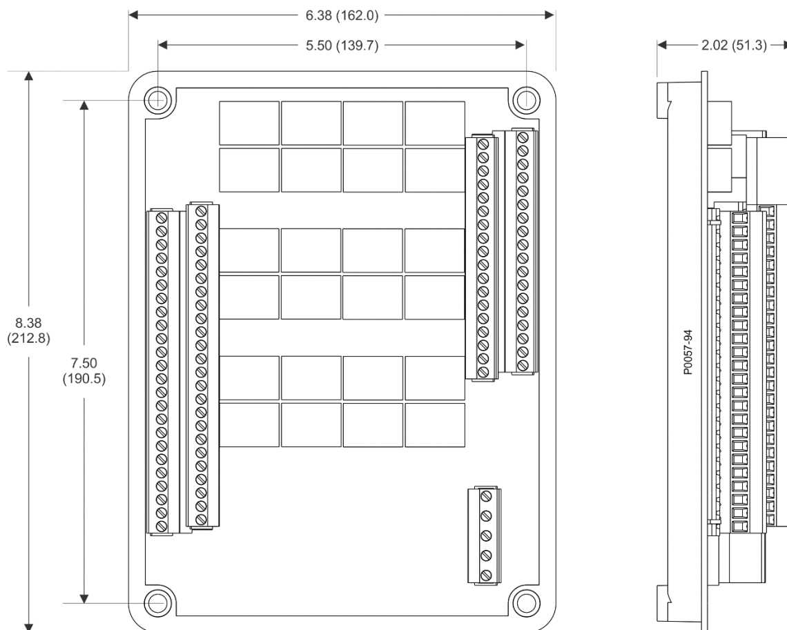
Figura 33-1. Dimensiones Generales del CEM-2020
