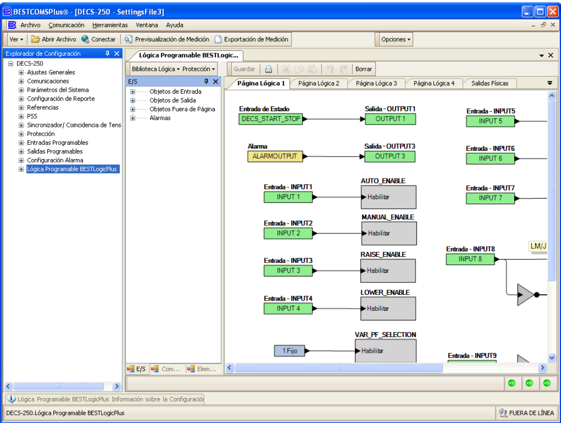
Figura 21-1. Esquema de Lógica Programable del BESTlogicPlus
