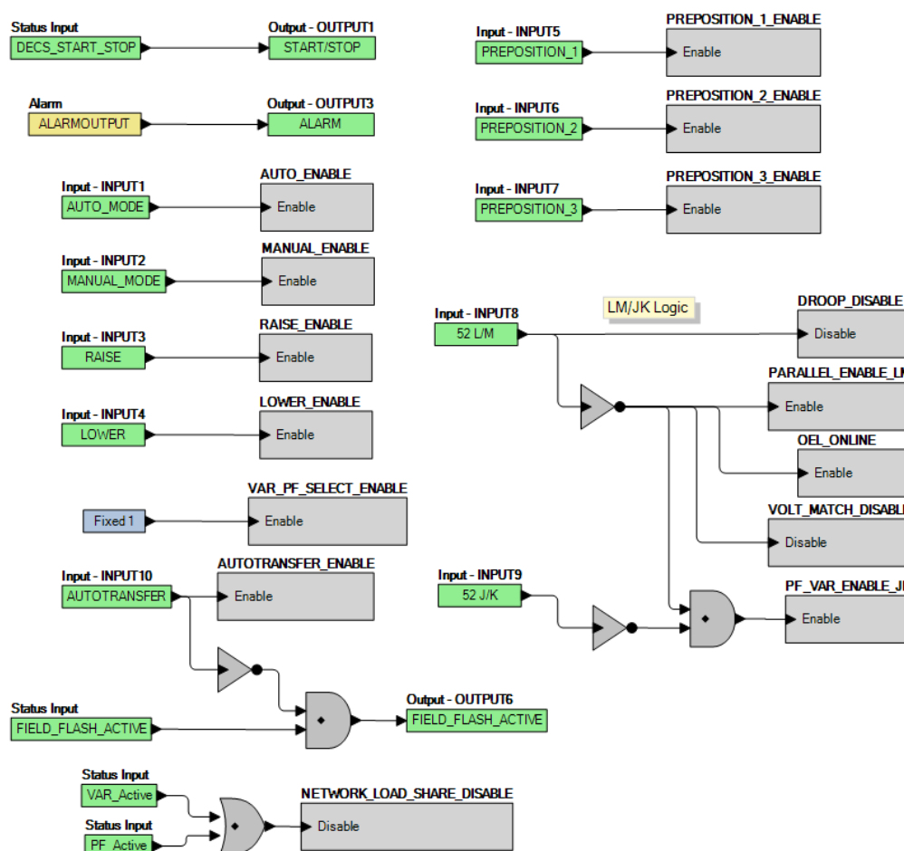
Figura 21-2. Lógica por Defecto del PSS Deshabilitado–1 Tab Página Lógica
