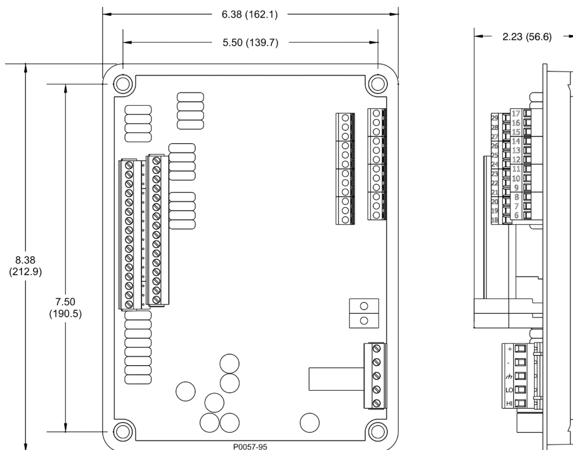
Figura 32-1. Dimensiones Generales del AEM-2020
