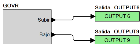
Figura 21-12. Ejemplo 1 - Conexiones del Bloque Lógico del GOVERNADOR
