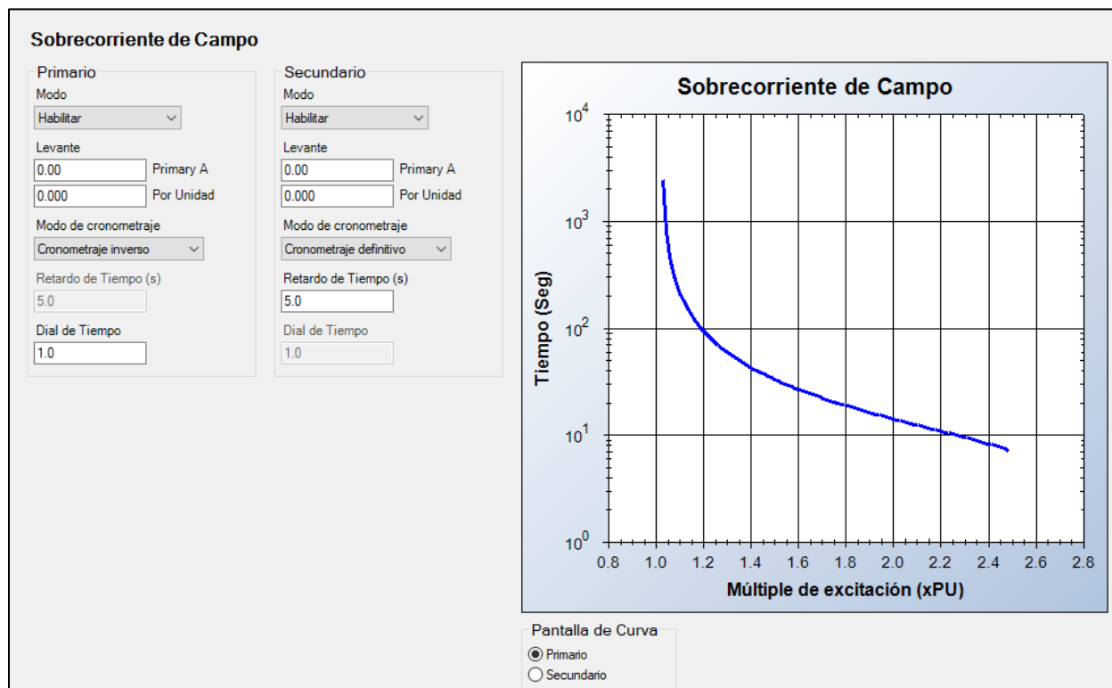
Figura 10-13. Ajustes de protección de sobrecorriente de campo
