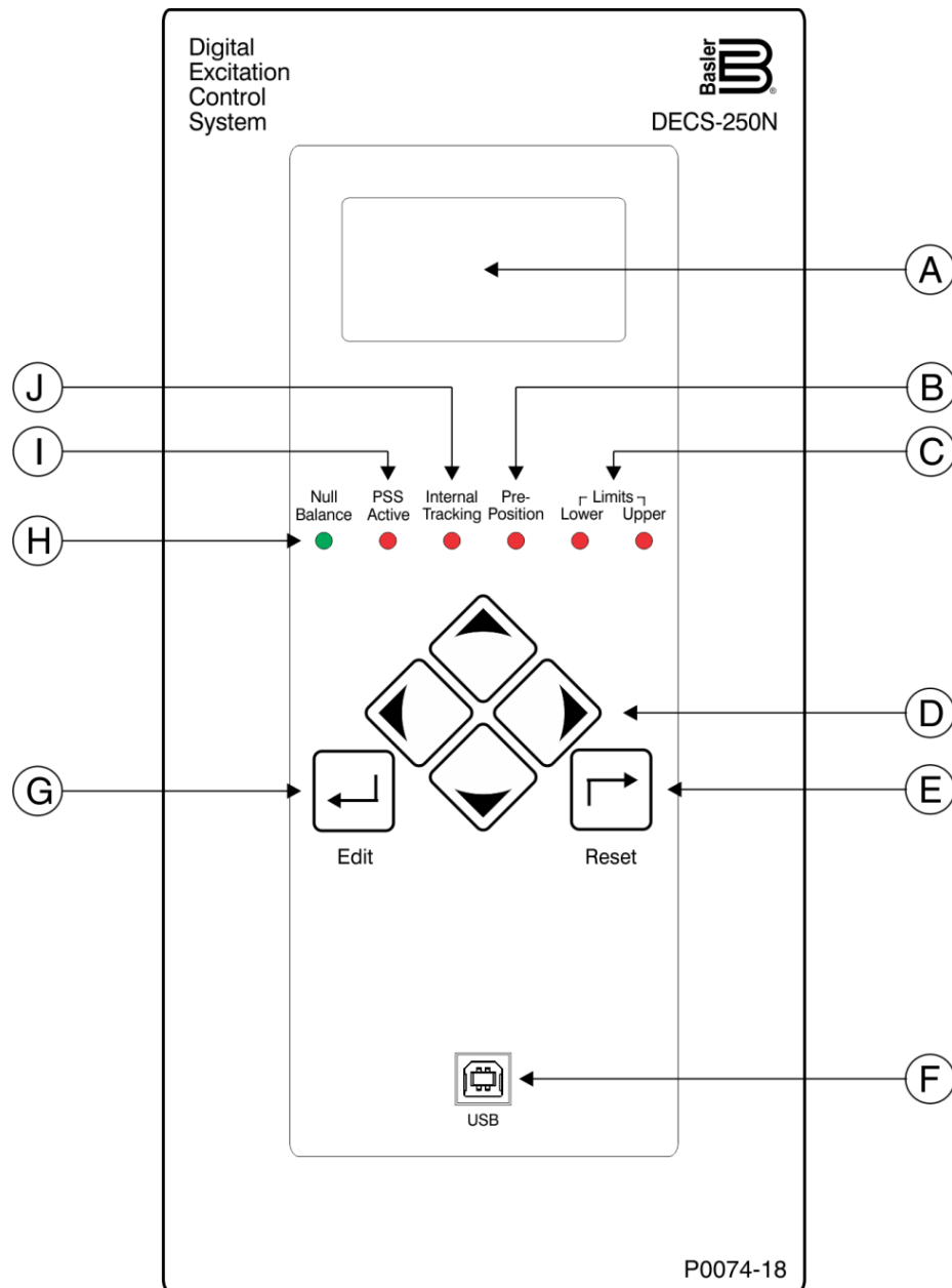
Figura 2-1. Controles e Indicadores del Panel Frontal
