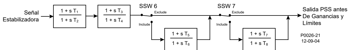
Figura 15-7. Compensación de Fase
