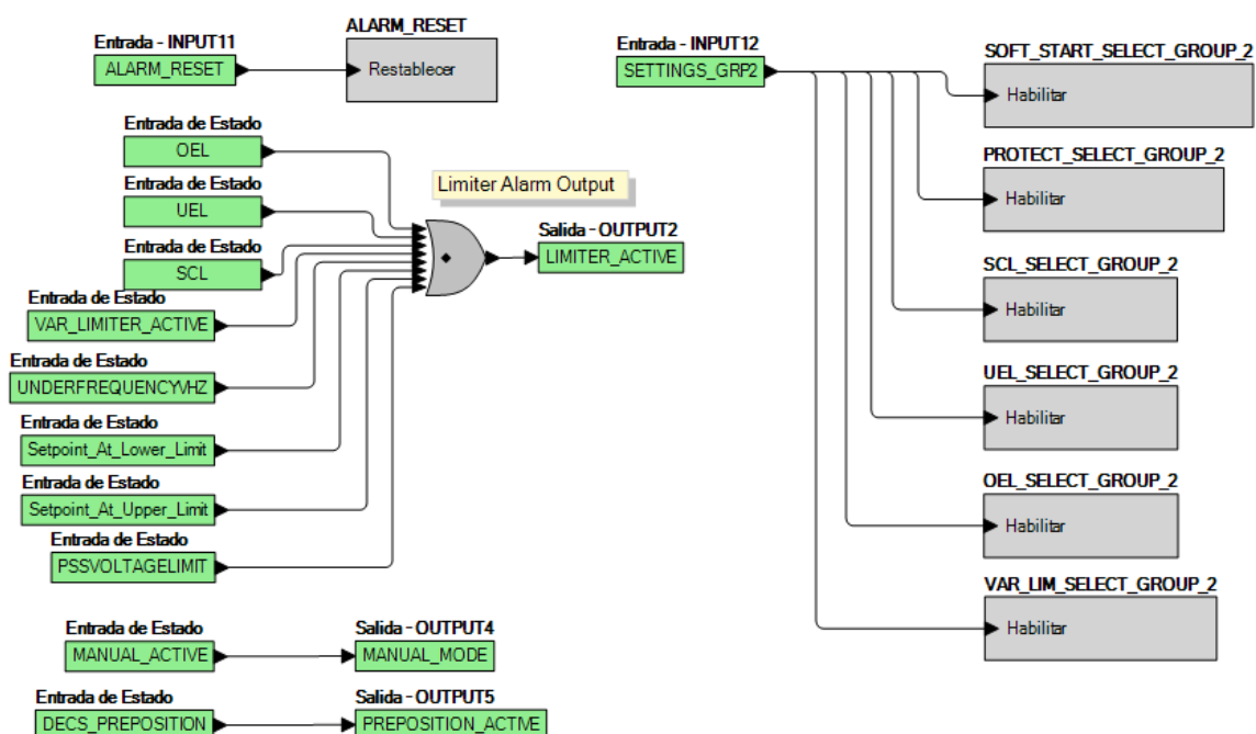
Figura 21-6. Lógica por Defecto PSS Habilitado - 1 Tab Página Lógica
