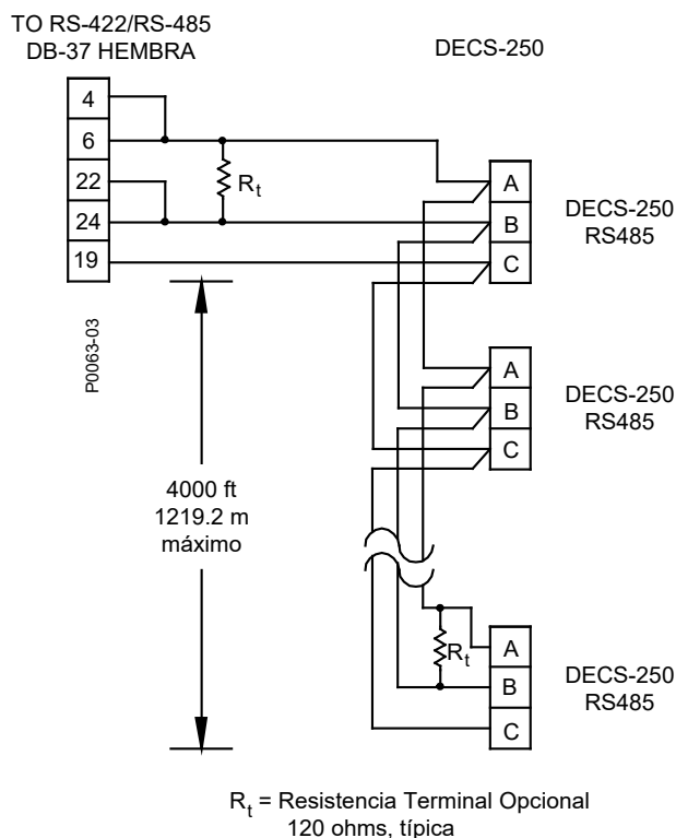
Figura 22-3. Conexiones Típicas del RS-485
