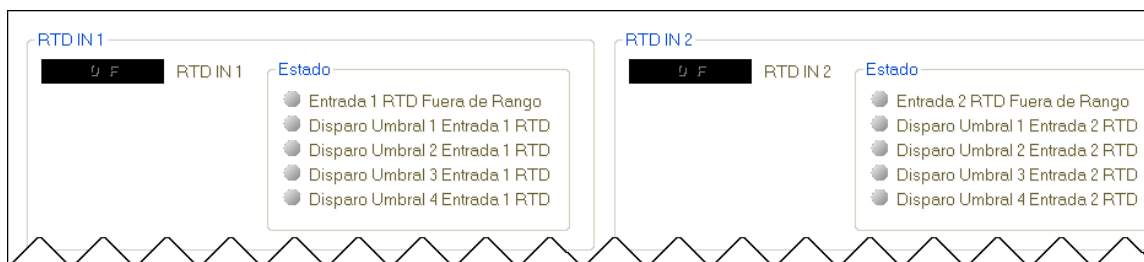
Figura 32-17. Medición de Entradas RTD Remotas
