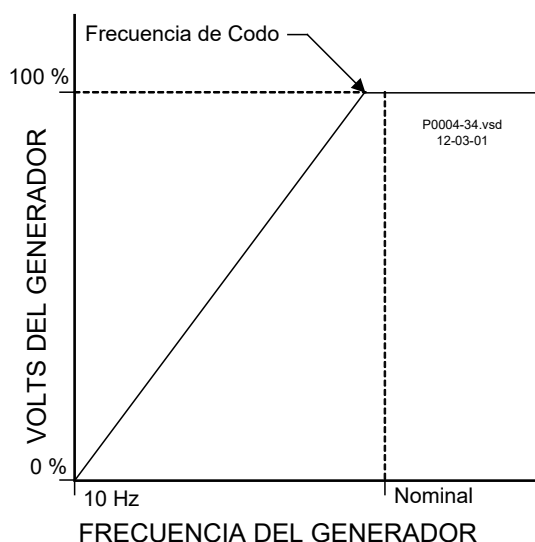
Figura 11-13. Curva de Compensación de Subfrecuencia Típica
