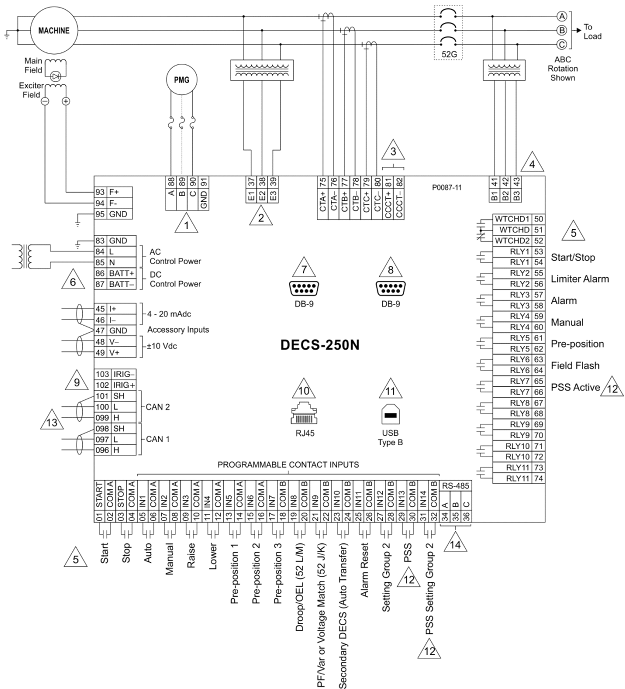
Figura 19-2. Conexiones de DECS-250N típicas para las aplicaciones accionadas por PMG
