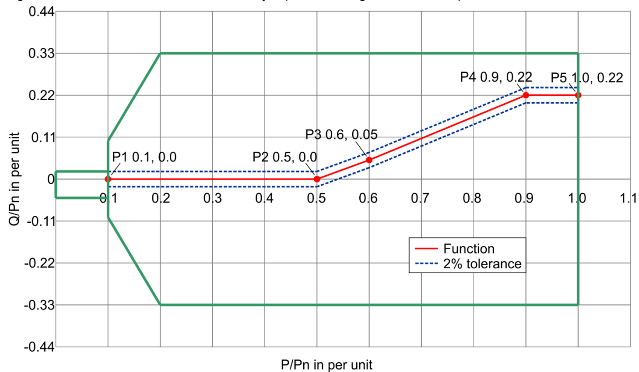
Figura 12-11. Ejemplo de Curva característica Q(P)
