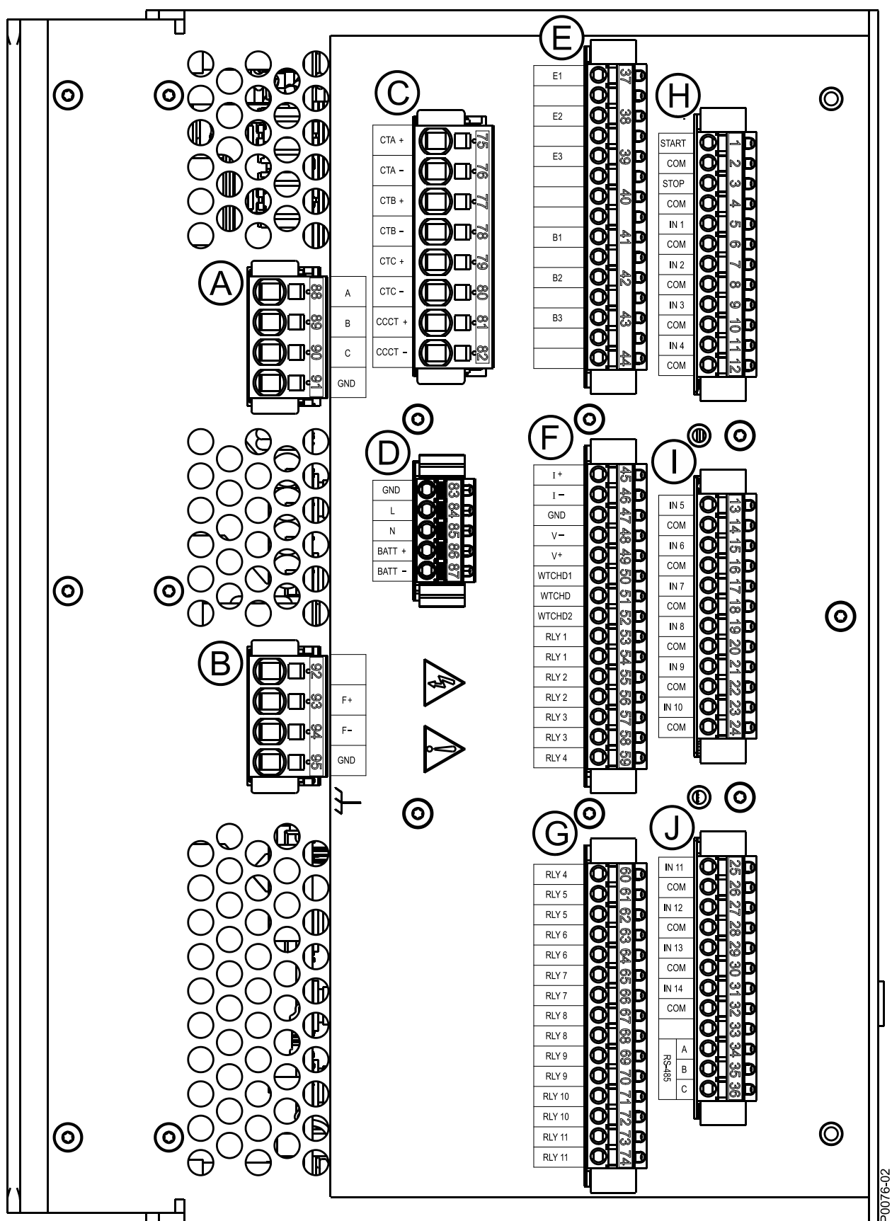
Figura 18-1. Terminales del panel izquierdo
