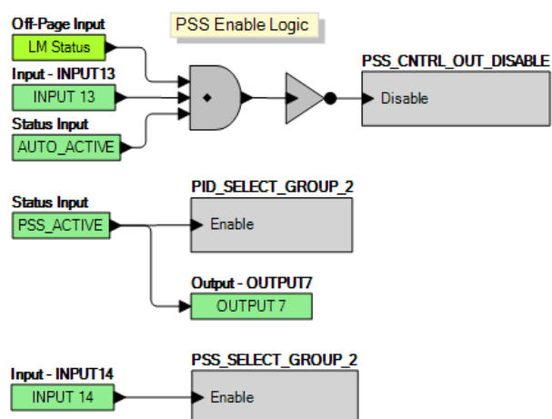
Figure 21-7. Lógica por Defecto PSS Habilitado - 3Tab Página Lógica
