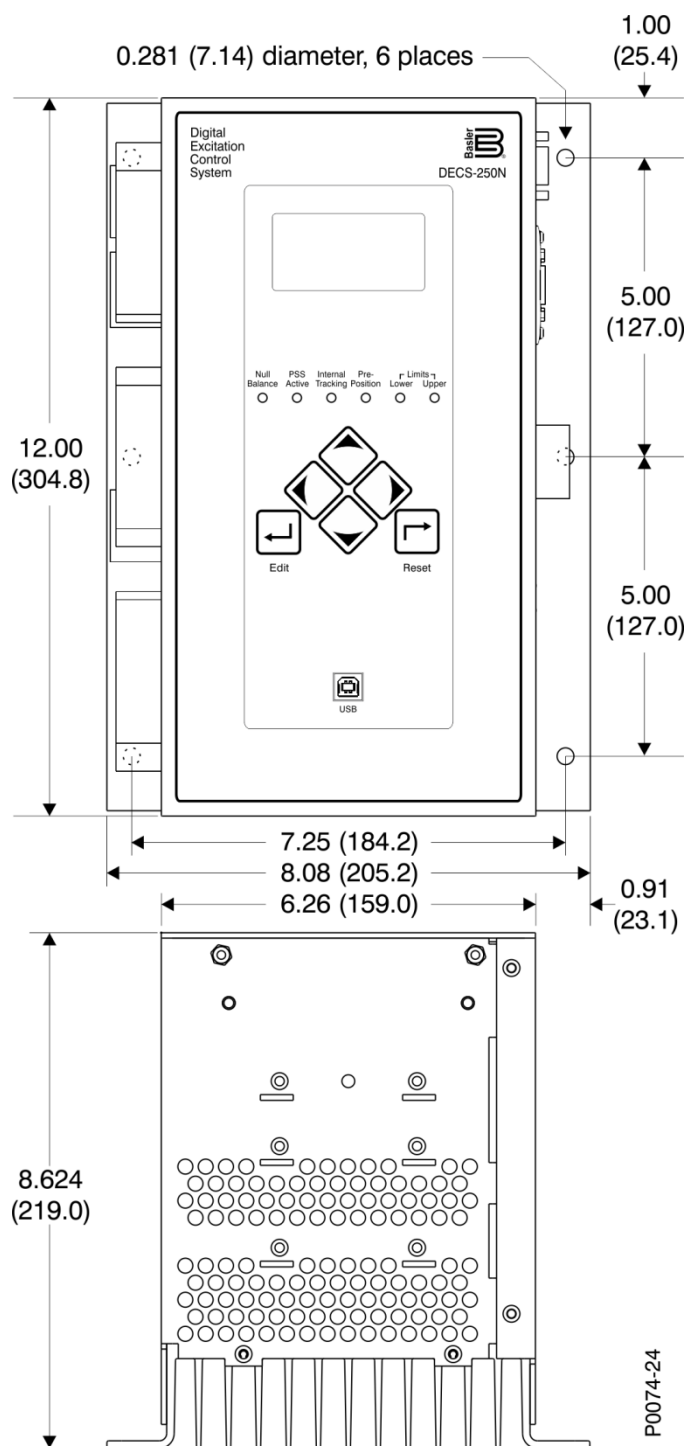
Figura 17-1. Dimensiones de Montaje Totales y de Proyección
