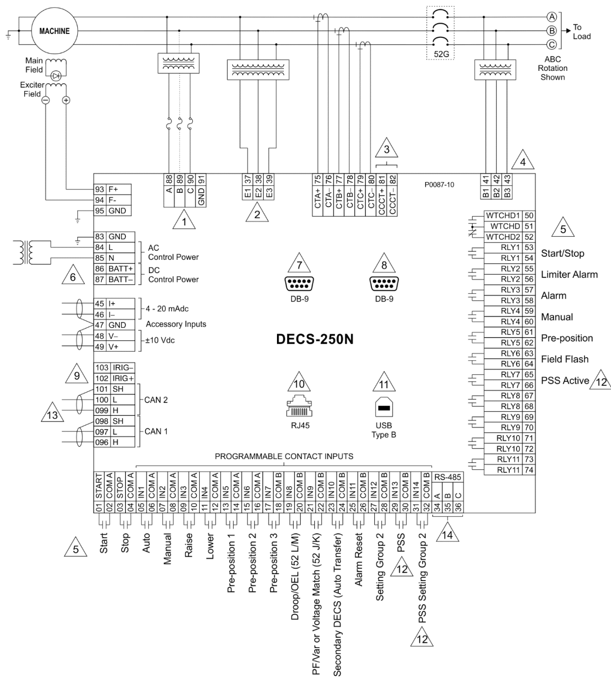
Figura 19-1. Conexiones de DECS-250N típicas para las aplicaciones accionadas por derivación
