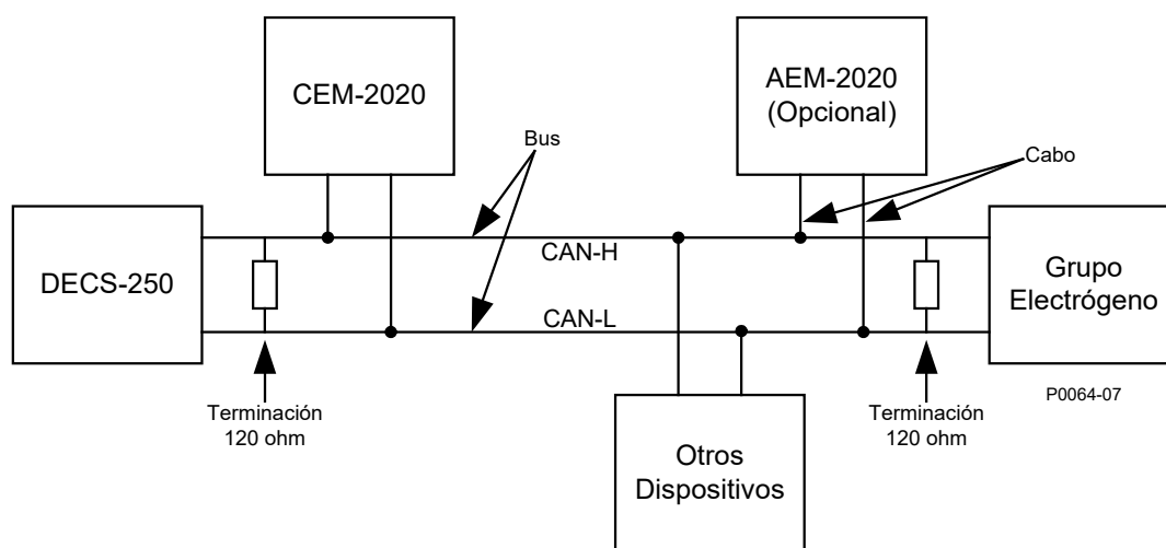
Figura 33-6. Interfaz del CAN Bus con el DECS-250N dando un Extremo del Bus
