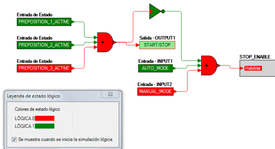
Figura 21-10. Ejemplo del simulador de lógica fuera de línea
