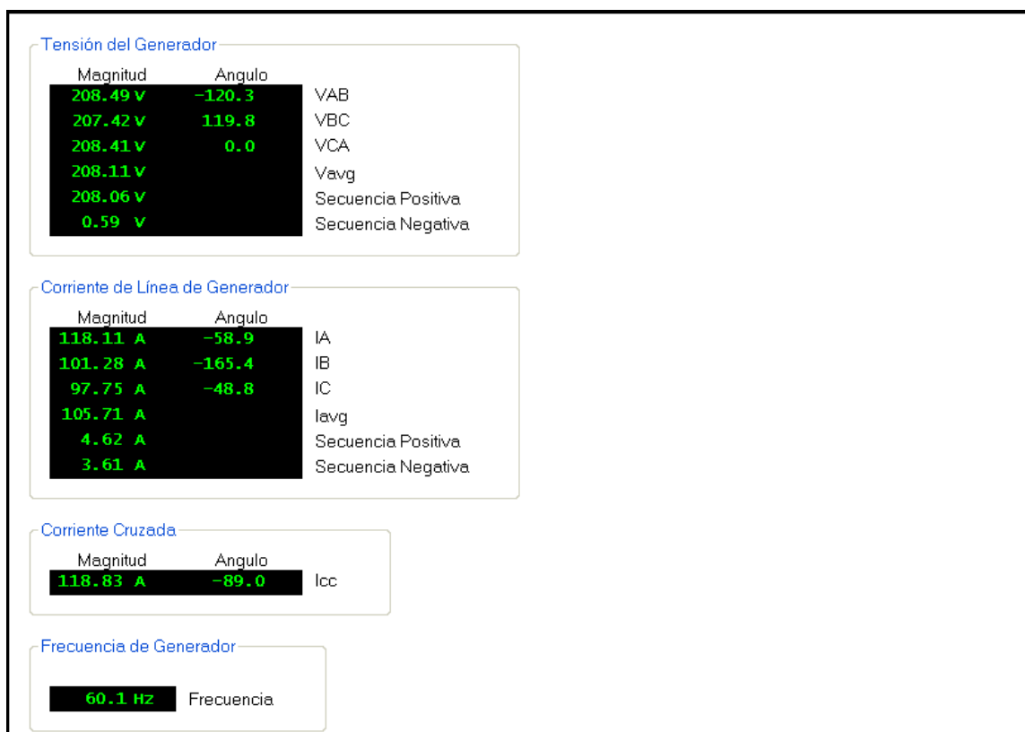
Figura 13-2. Medición de los Valores Primarios del Generador
