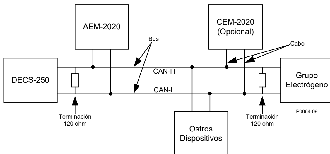
Figura 32-10. Interfaz de CAN Bus con DECS-250N proporcionando Un Extremo del Bus
