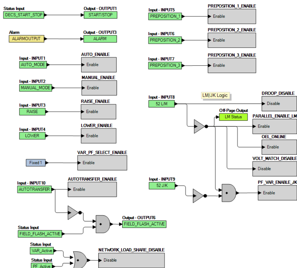
Figura 21-5. Lógica por Defecto del PSS Habilitado- 1 Tab Página Lógica
