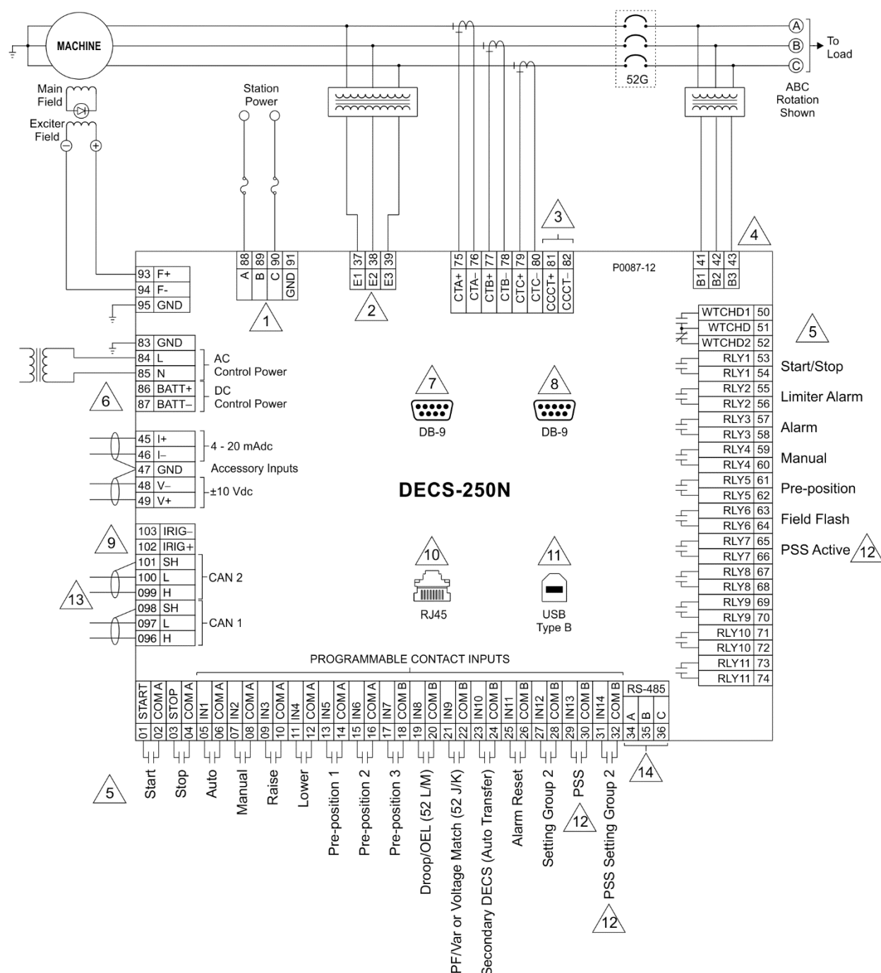
Figura 19-3. Conexiones de DECS-250N típicas para las aplicaciones accionadas en la estación
