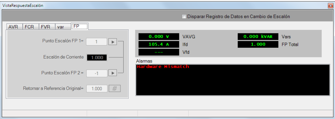
Figura 26-5. Análisis de Respuesta de Escalón –Tab PF
