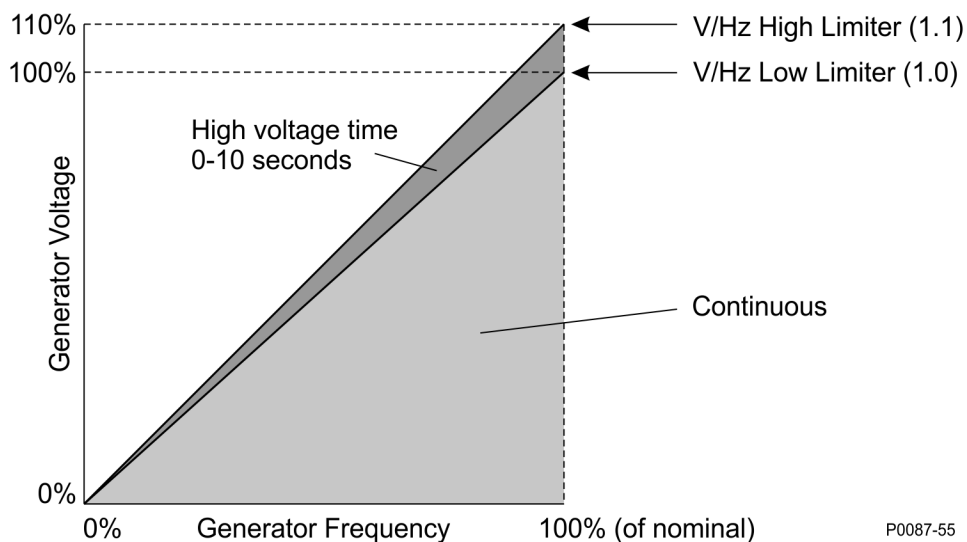
Figura 11-14. Curva de Limitador 1.1 PU Volts por Hertz Típica
