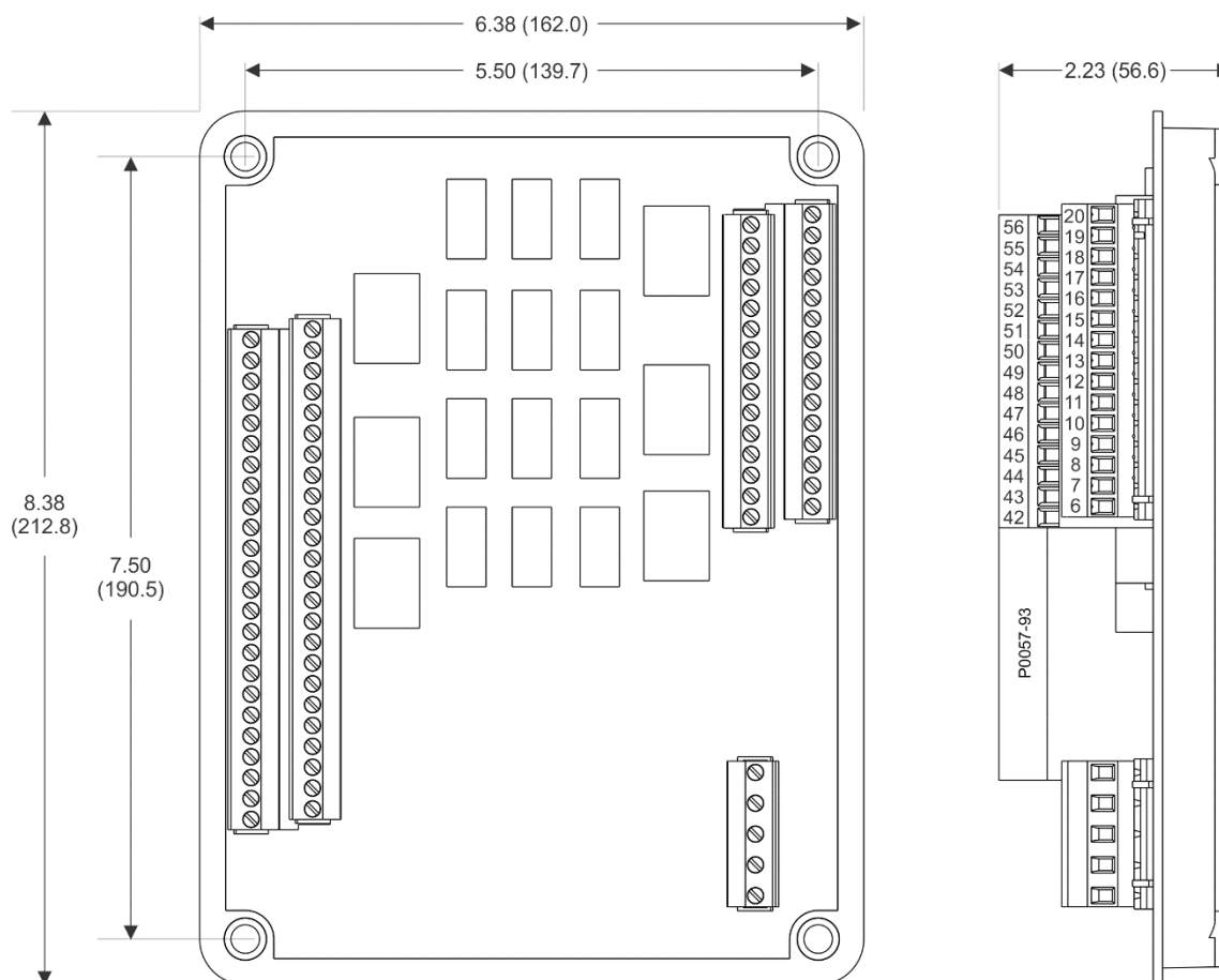
Figura 33-2. Dimensiones Generales del CEM-2020H
