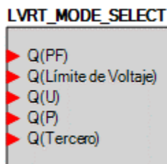
Figura 12-12. Elemento lógico de Selección de modo LVRT
