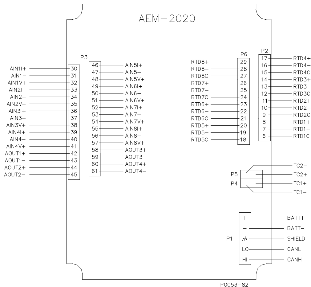
Figura 32-2. Terminales de Entrada y Salida
