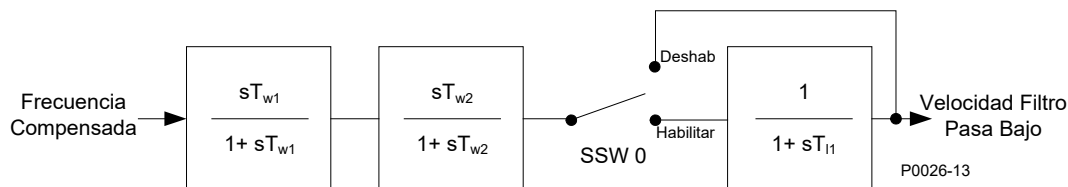
Señal de Frecuencia de Entrada PSS
