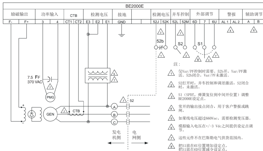
图2 - BE2000E 典型接线带三相检测
