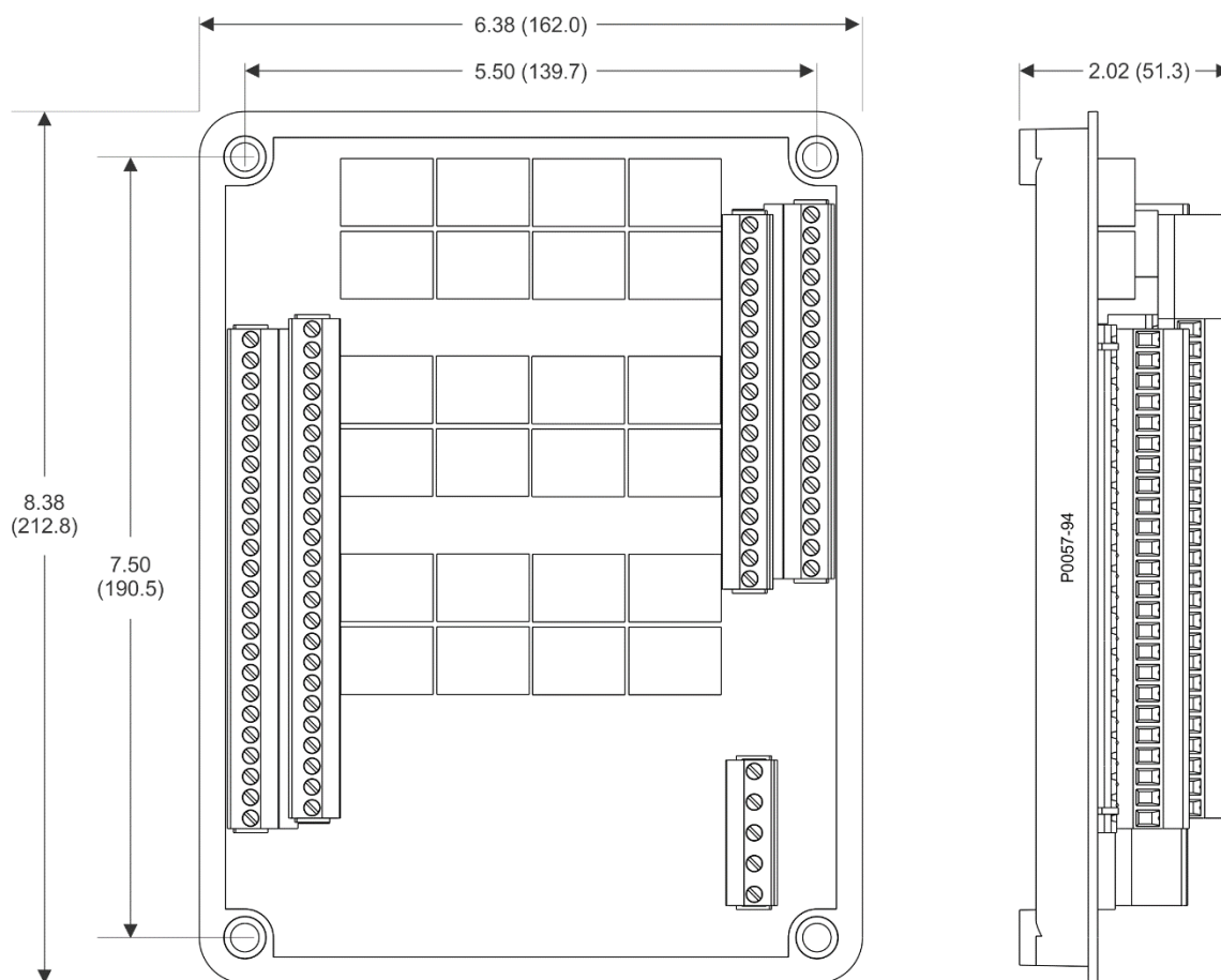
Figura 31-1. Dimensiones generales del CEM-2020
