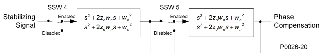
Figura 13-5. Filtros torsionales
