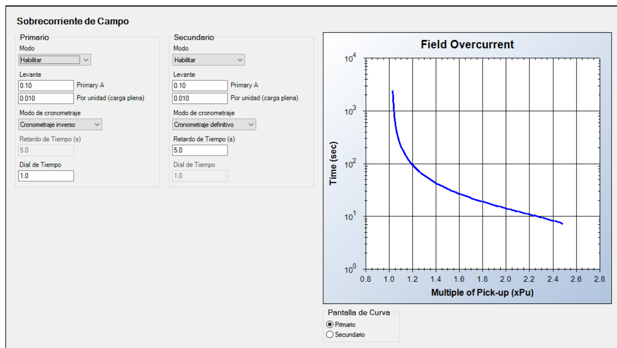
Figura 9-13. Ajustes de la protección de sobrecorriente de campo
