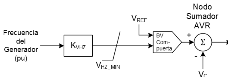
Figura 33-21. Limitador de Voltios por Hercio
