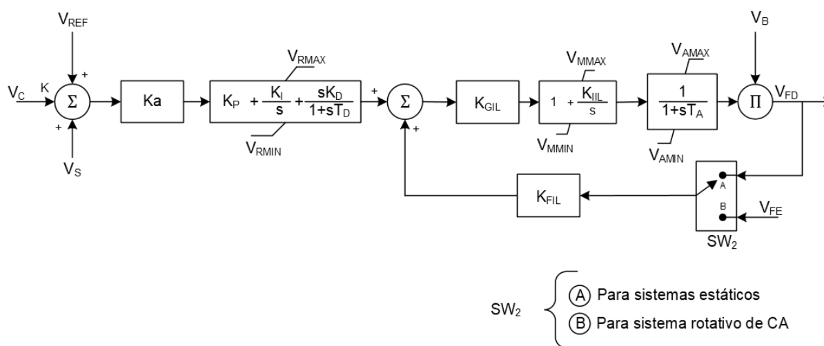
Figura 33-6. Diagrama de Bloques del AVR por Unidad con Regulador de Campo de Bucle Interno
