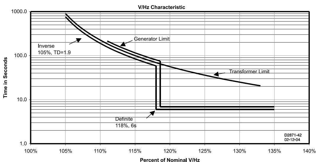
Figura 9-1. Característica de V/Hz - El tiempo se muestra en el eje vertical
