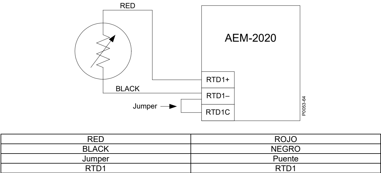
Figura 30-7. Conexiones de entradas de RTD bifilares externas
