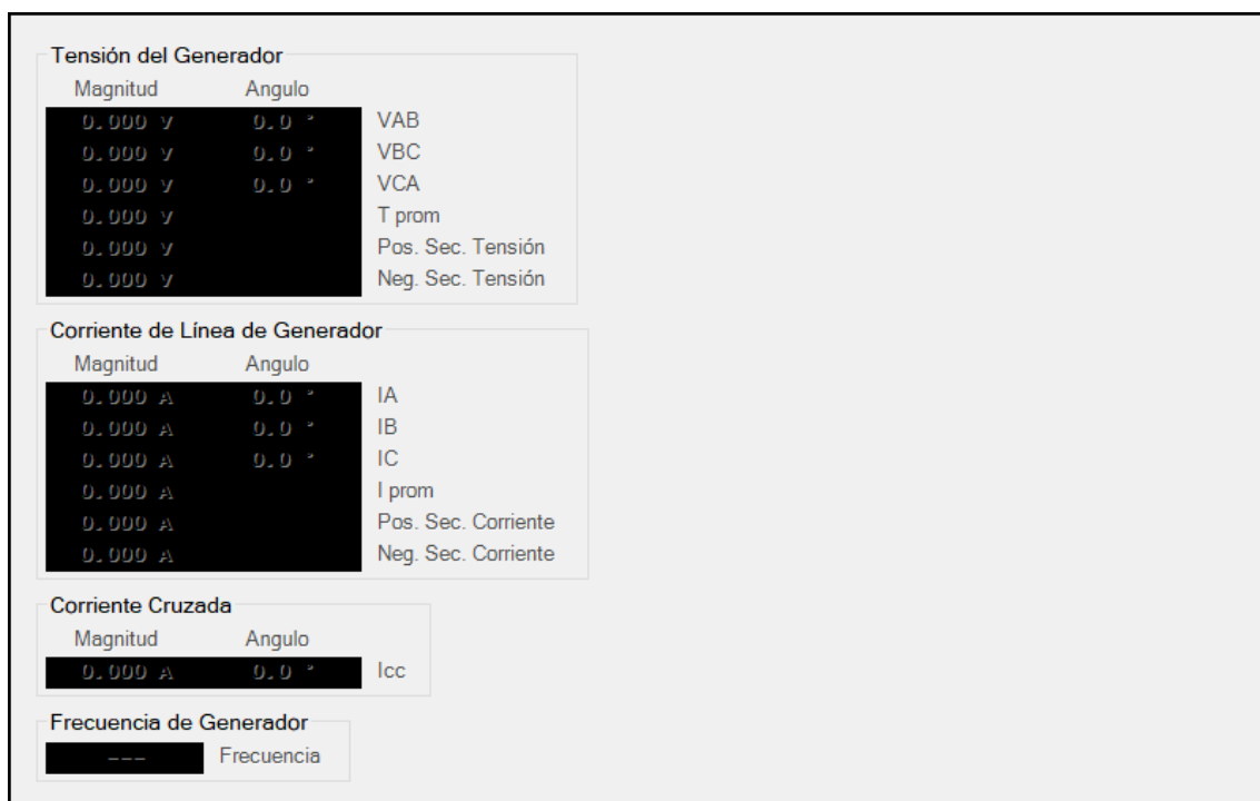
Figura 11-2. Medición de valores primarios del generador
