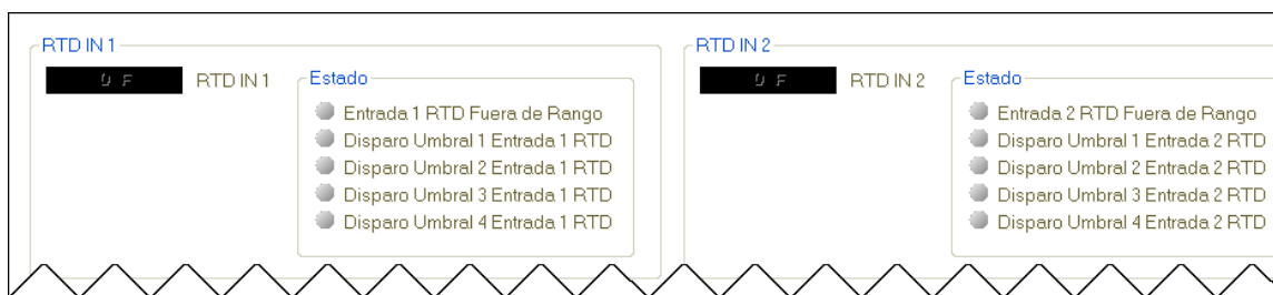
Figura 30-17. Medición de las entradas de RTD remotas
