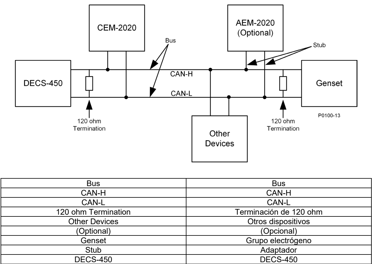
Figura 31-4. Interfaz de bus CAN con DECS-450 que proporciona un extremo del bus
