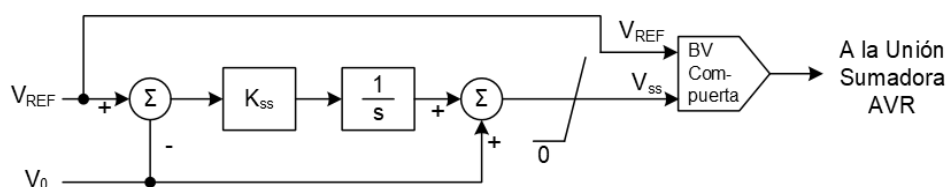
Figura 33-23. Diagrama de Bloques de Control de Arranque Suave por Unidad
