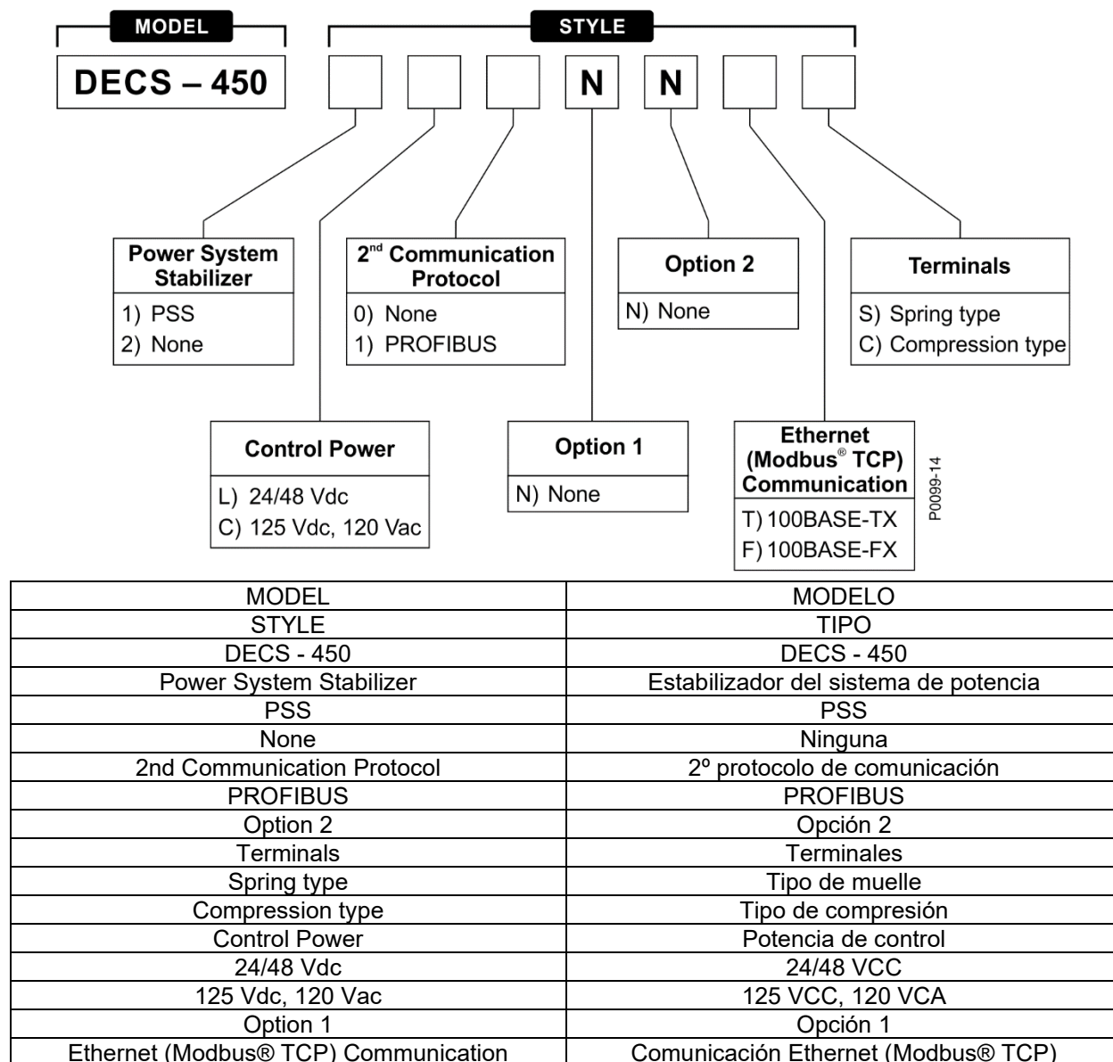
Figura 1-1. Gráfica de tipo del DECS-450
