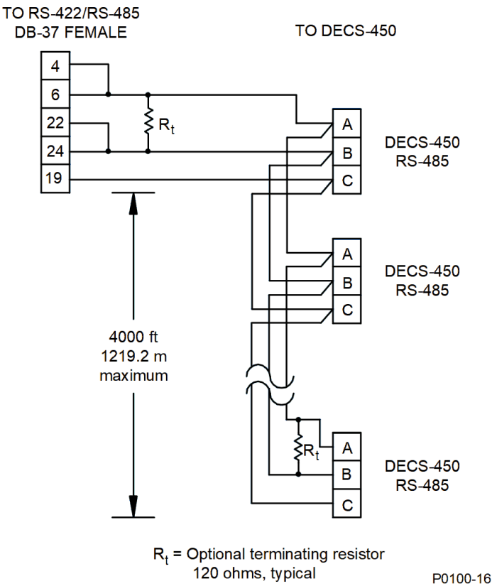
Figura 20-2. Conexiones RS-485 típicas
