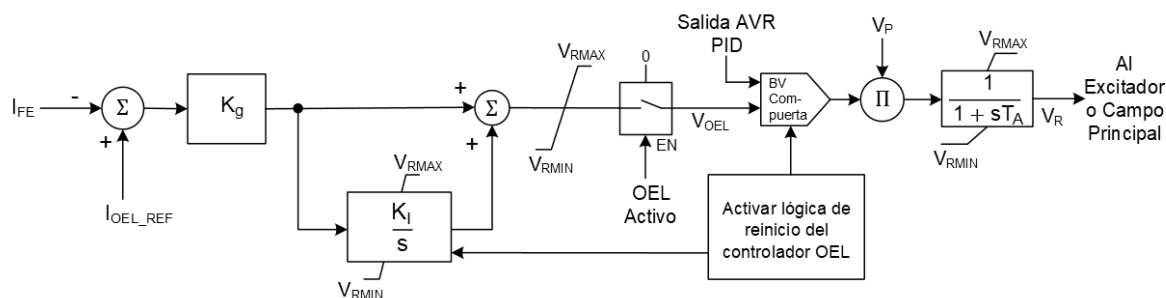
Figura 33-15. Diagrama de Bloques del Limitador de Sobreexcitación de tipo Toma de Control por Unidad
