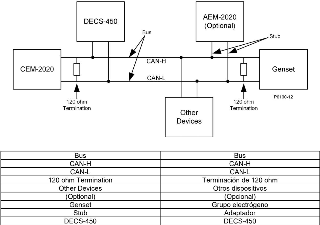
Figura 31-3. Interfaz del bus de la CAN con el CEM-2020, que brinda un extremo del bus
