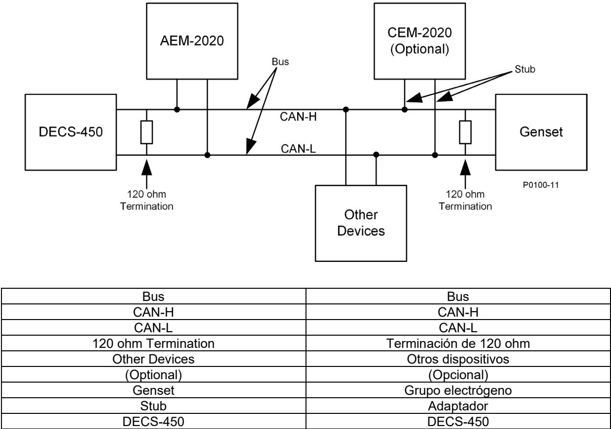
Figura 30-10. Interfaz de bus CAN con DECS-450 que proporciona un extremo del bus
