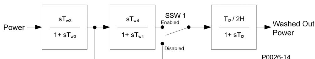
Figura 13-2. Señal de potencia eléctrica del generador
