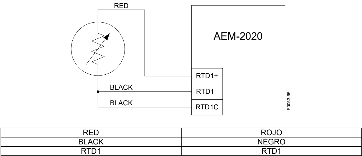
Figura 30-8. Conexiones de entradas de RTD trifilares externas
