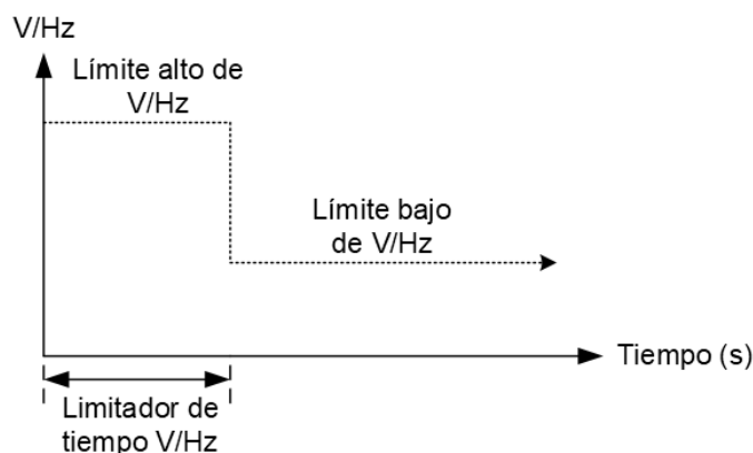
Figura 33-20. Selección de Pendiente de Voltios por Hercio
