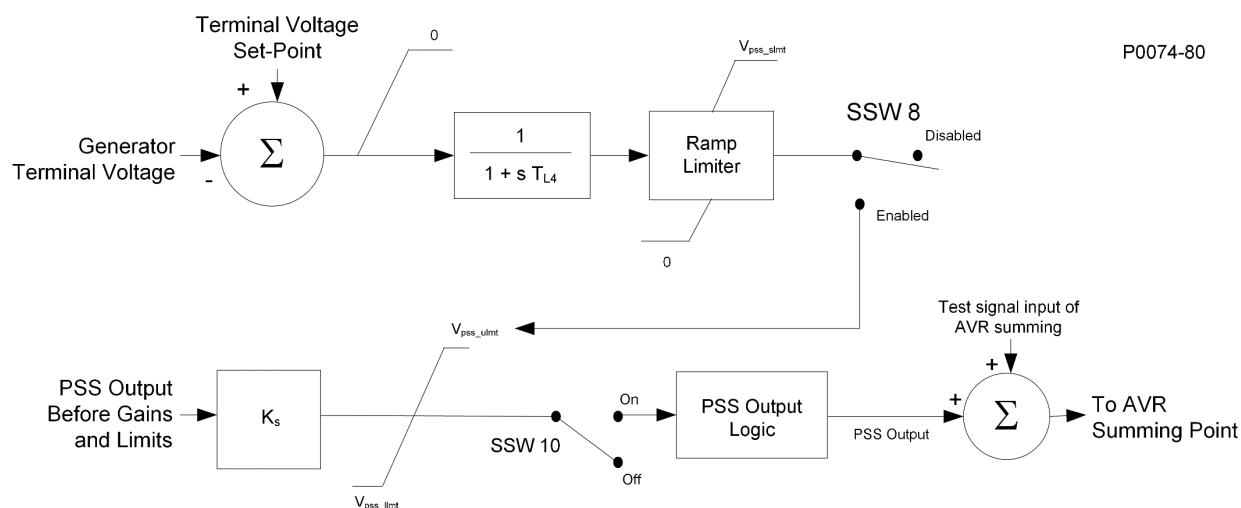
Figura 13-8. Etapa de salida
