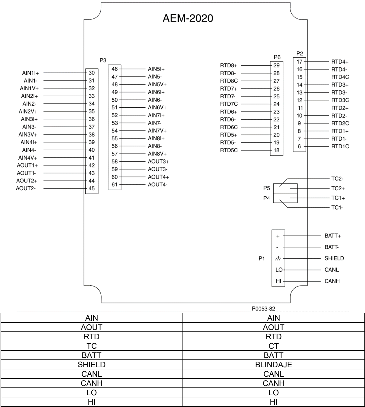
Figura 30-2. Terminales de entrada y salida
