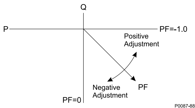
图 12-19. 功率因数：负
