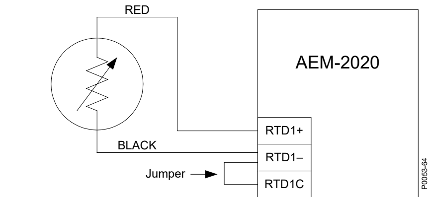
图 32-7. 外部 2-线 RTD 输入连接
