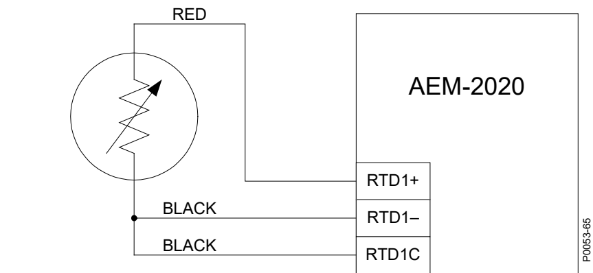
图 32-8. 外部 3-线 RTD 输入连接
