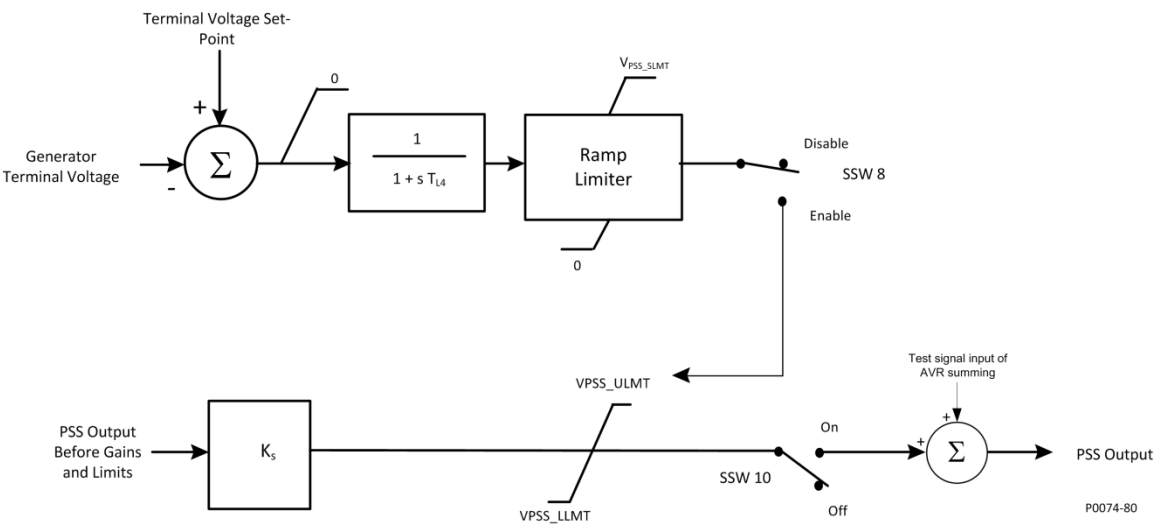
图 15-9. 输出等级
