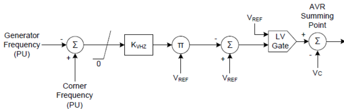
图34-15. 低频限制器
