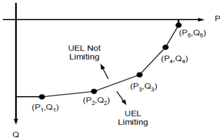
图34-9. 用固定图的五点 UEL 曲线特性
