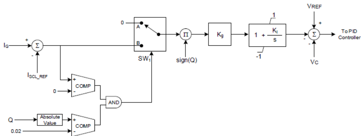
图34-13. 求和点型定子限流器的每元框
