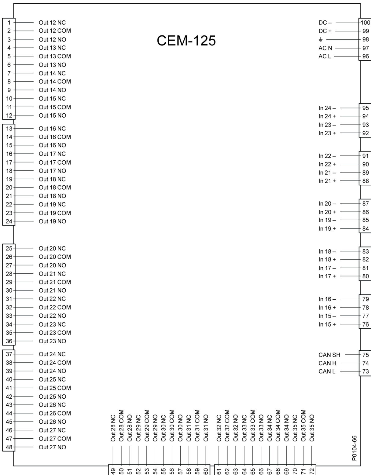
Abbildung 5-1. CEM-125-Anschlüsse
