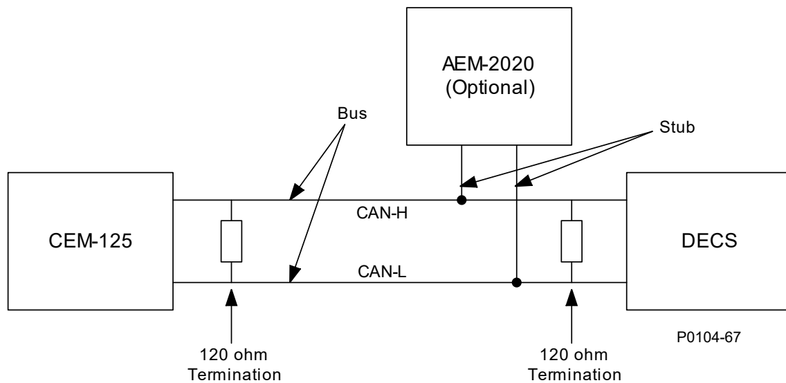
Abbildung 5-3. CAN-Bus-Schnittstelle mit CEM-125 Bereitstellung eines Endes des Busses
