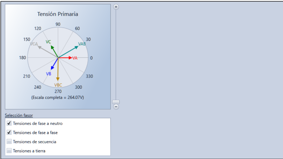
Figura 53-3. Pantalla de medición de fasores de tensión primaria
