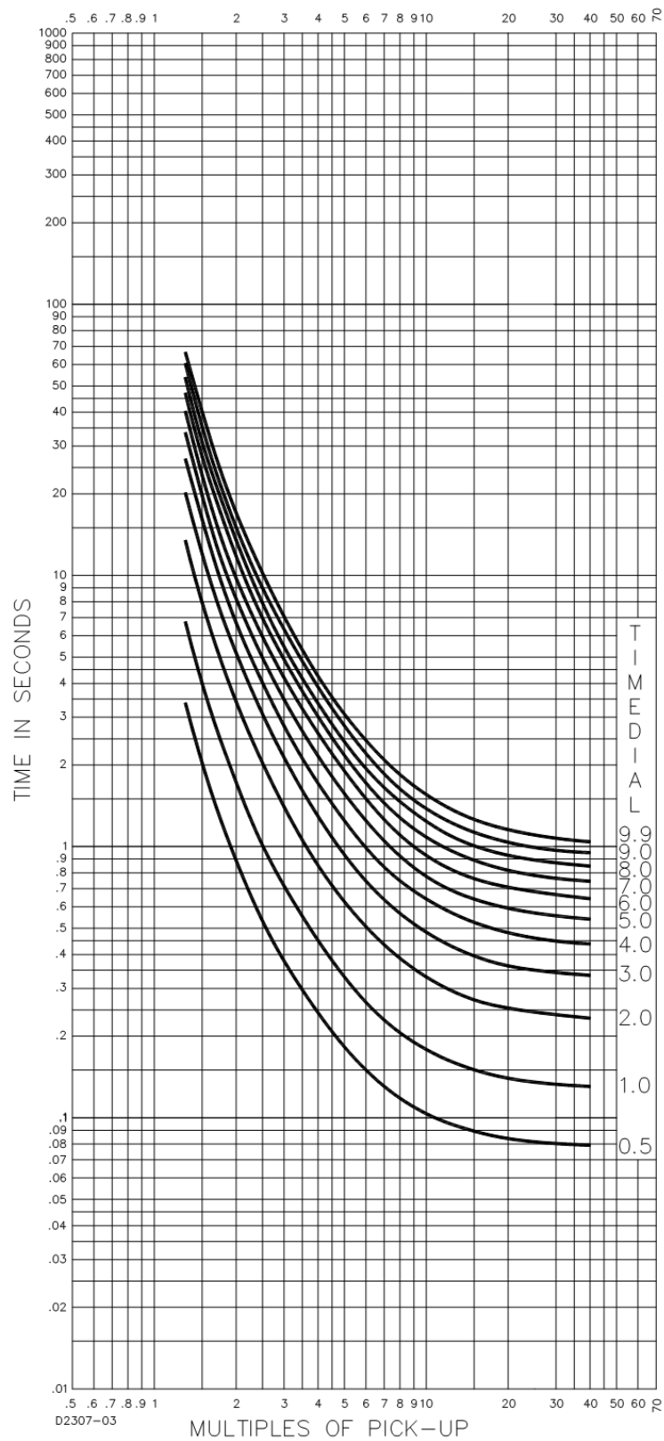
Figura 58-17. Curva de características de tiempo V2, muy inversa (similar a GE IAC-53)
