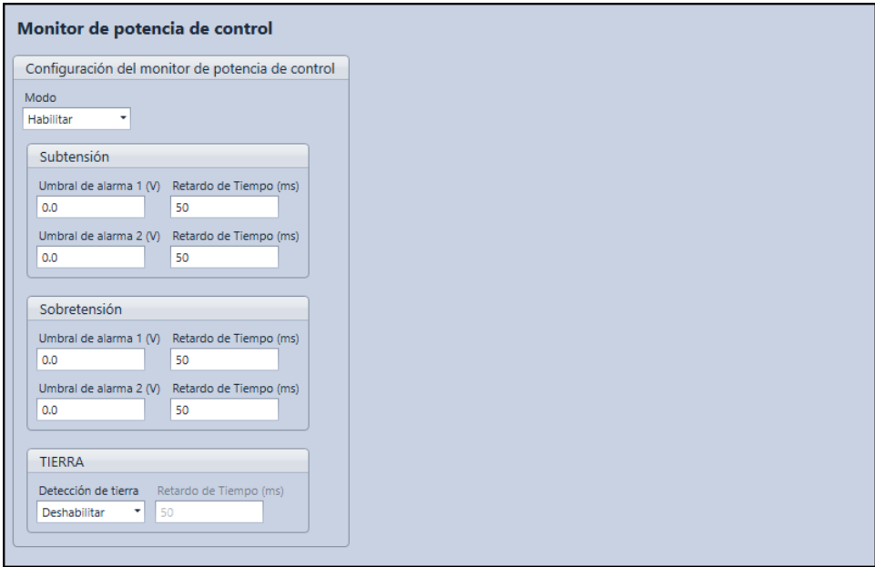
Figura 42-2. Pantalla de ajustes del Monitor de potencia de control
