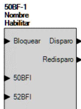
Figura 28-2. Bloque lógico del elemento falla del cortacircuitos
