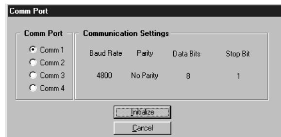
Figura5-4. Pantalla de inicio de comunicación
