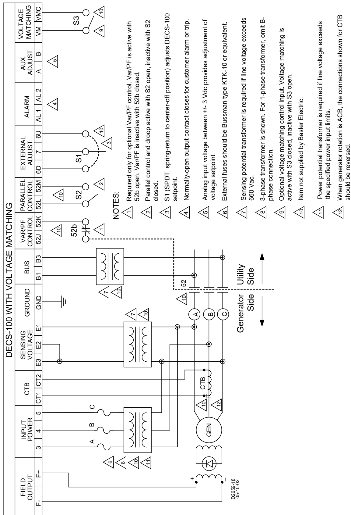
Figura4-9. Conexiones típicas para aplicaciones de derivación con rotación ABC y detección monofásica
