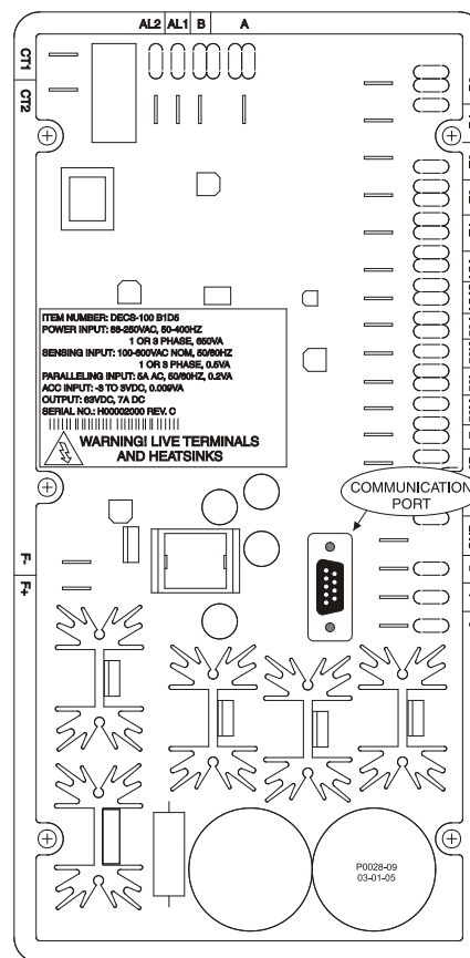
Figura2-2. DICS-100 Ubicación del puerto de comunicación
