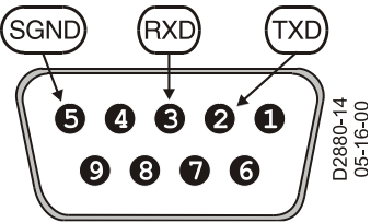
Figura4-4. Asignaciones de pines de puerto RS-232
