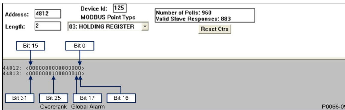
Figure 1-3. 32-Bit Bit-Mapped Parameter Mapping
